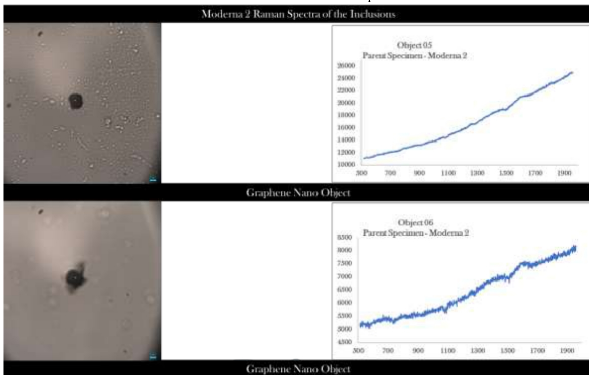
Figura 3.18. Espectros Raman de varias inclusiones en Moderna 02.
